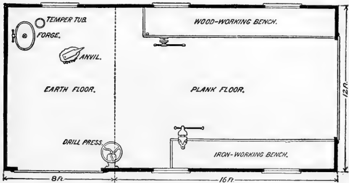
FIG. 234.—Floor plan of workshop. (U. S. D. A.)
